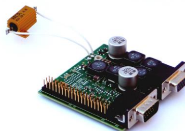
QCI-S2-IG-01
