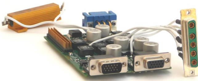
QCI-S3-IG-01
