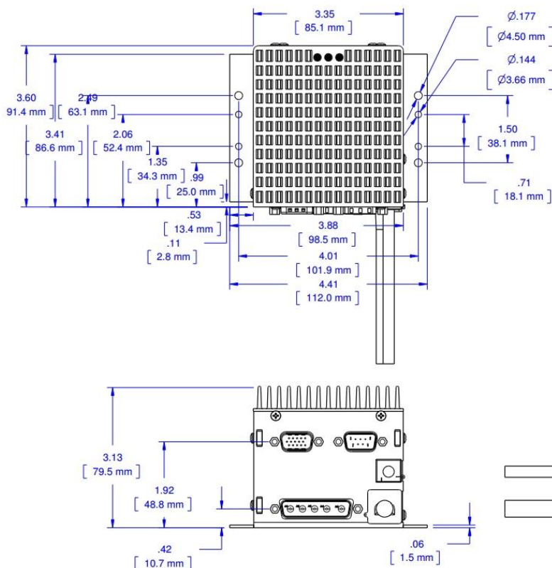
QCI-N3-MX Mechanical
