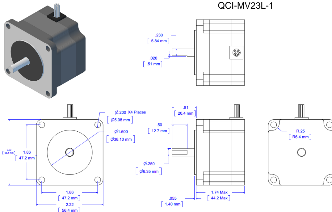
QCI-MV23L-1
